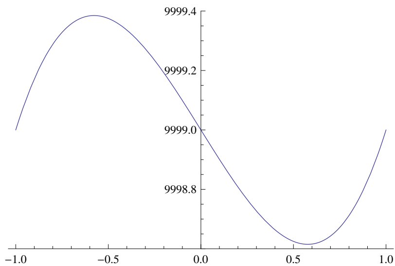
図 1: 三次関数のグラフ
