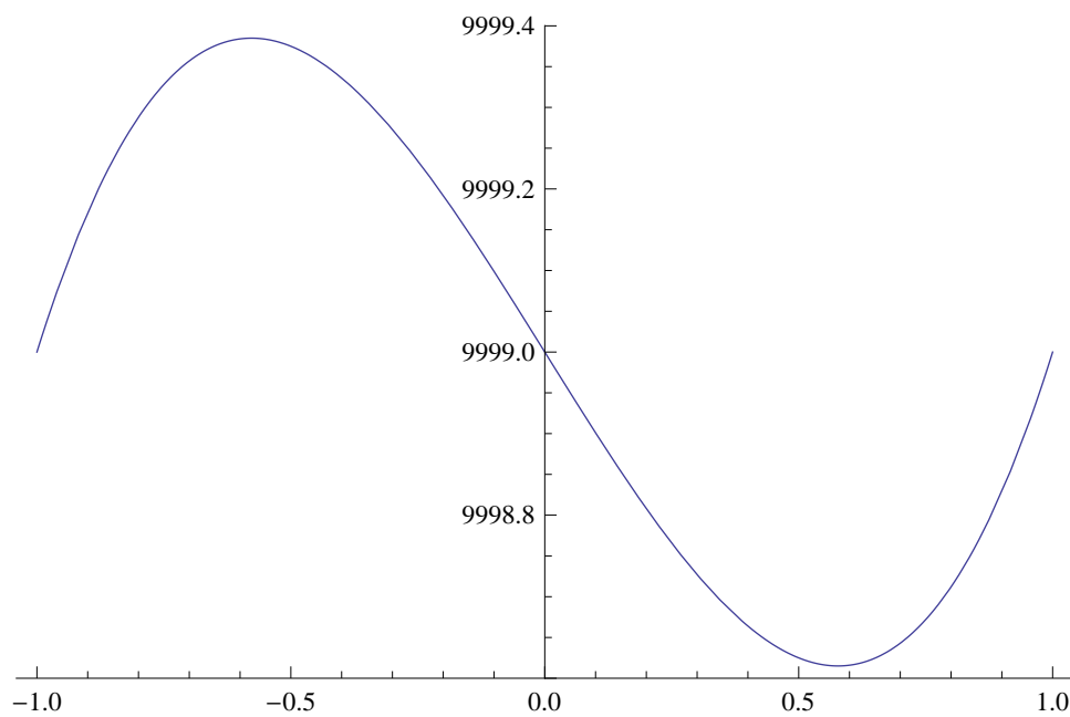
図 1: 三次関数のグラフ
